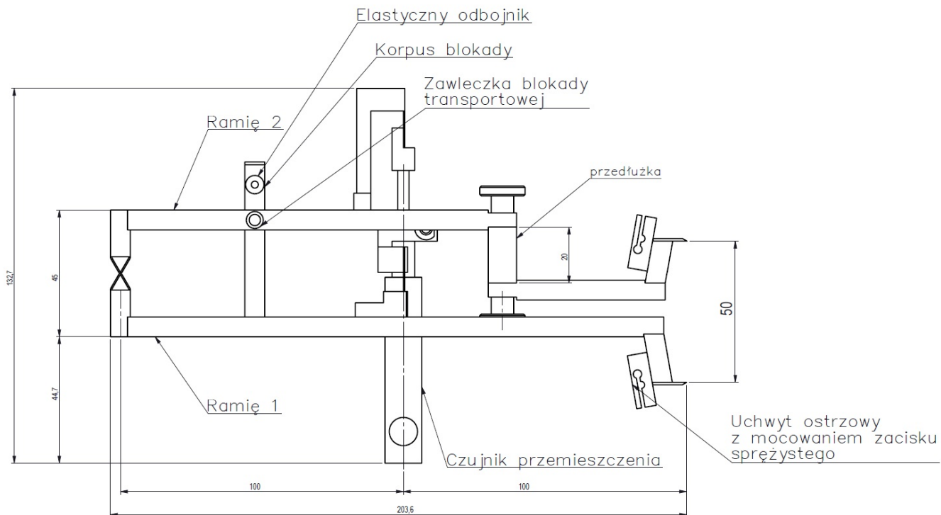
Rys. 1 Elementy składowe ekstensometru z zaznaczeniem gabarytów i wymiarów istotnych z punktu widzenia własności użytkowych (przedstawiona konfiguracja bez płytek dystansowych w wartości początkowej długości pomiarowej L_0=100\text{mm} ).
